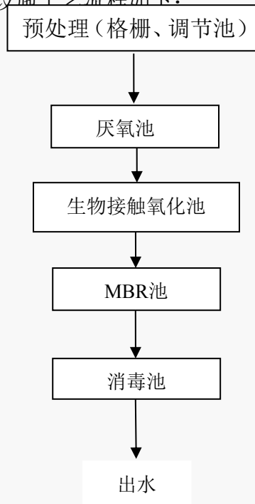
图3-3 污水处理工艺图
